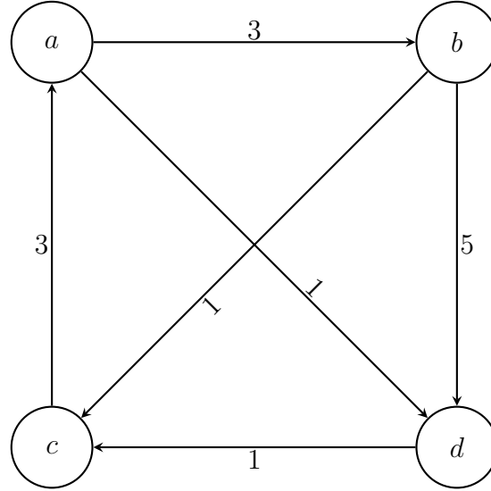
Figure 2.5: Graf otrzymany po dodaniu głosu typu abcd
