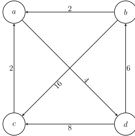
Figure 2.6: Graf otrzymany po dodaniu głosu typu dcba
