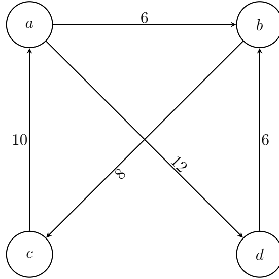
Figure 2.4: Graf większościowy dla profilu R^V
