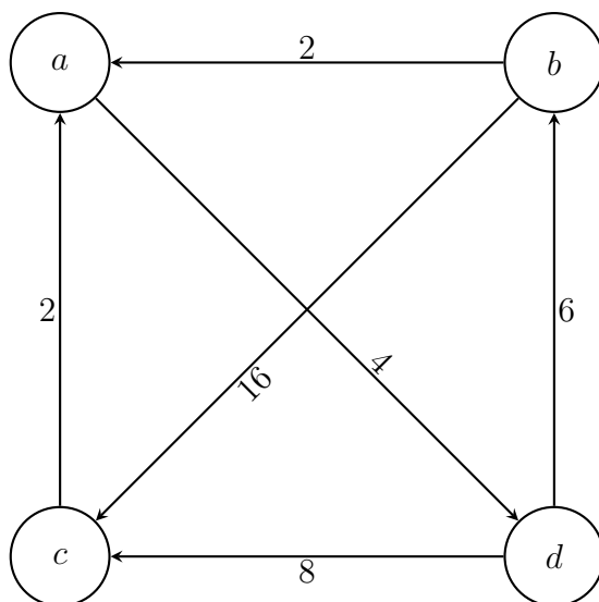
Figure 2.3: Graf większościowy dla profilu R^W
